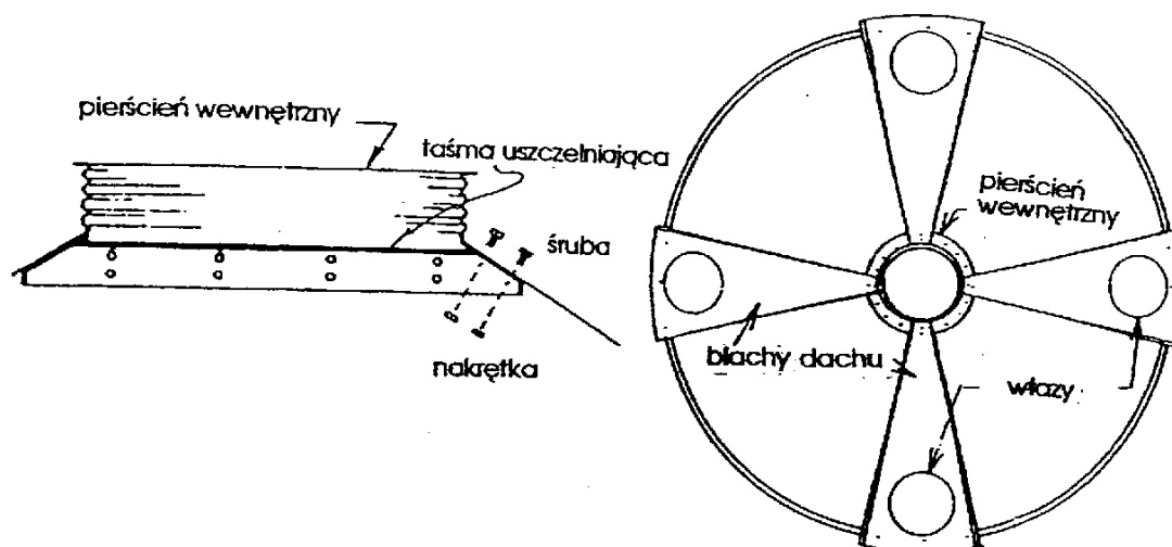
Widok czterech (4) płyt dachowych opartych na pierścieniu wewnętrznym (zworniku) i pierścieniu zewnętrznym
